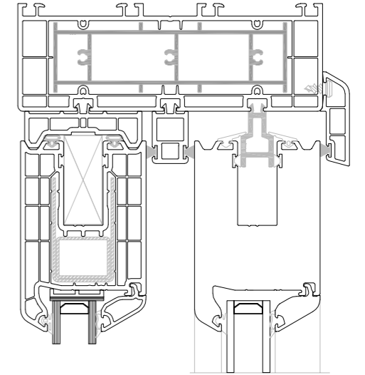
D-DETAYI
