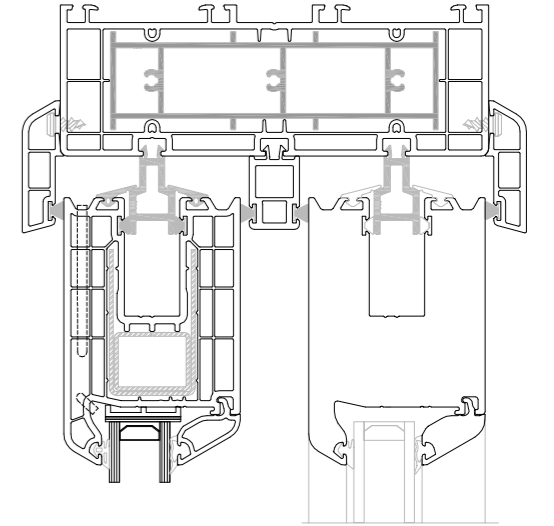
D-DETAYI
