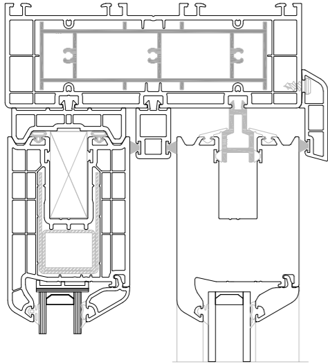
A-DETAYI
