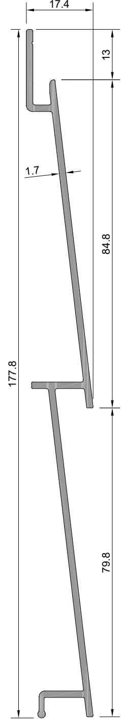
Profil No: COT-209 Ağırlık : 1038 gr/m
