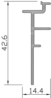
Profil No: D2-501 Ağırlık : 232 gr/m
