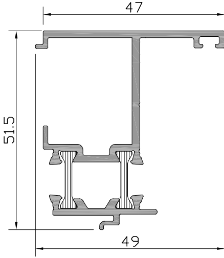
Profil No: D1-501
