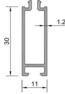
Profil No : KC0331 Ağırlık : 209 gr/m
